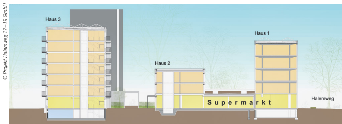
Giebelansicht der Häuser 1–3 (Blick vom Grünzug Popitzweg–Halemweg). Zwischen den Häusern 2 und 3 ist ein direkter Durchgang zum U-Bahnhof und zum Grünzug geplant. Der Supermarkt befindet sich künftig im Erdgeschoss von Haus 1 und 2.
